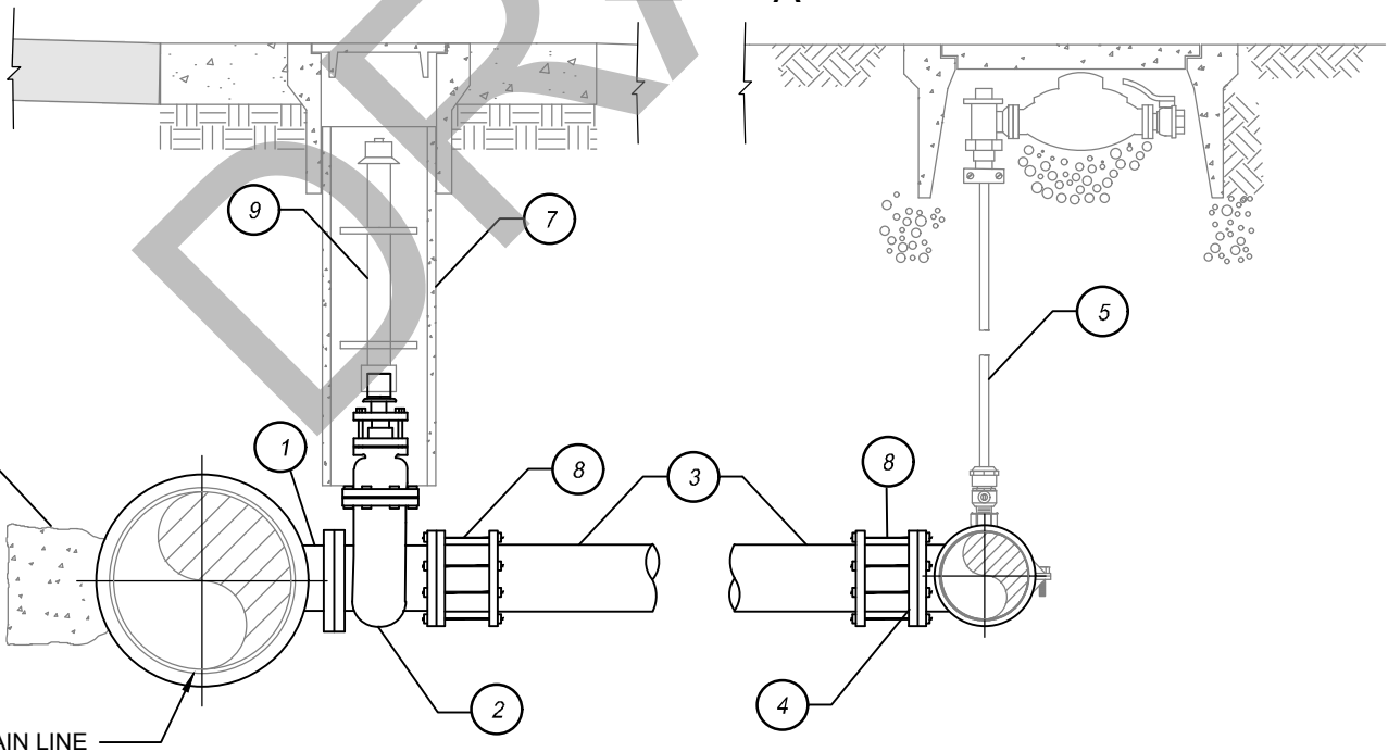
SECTION A-A
