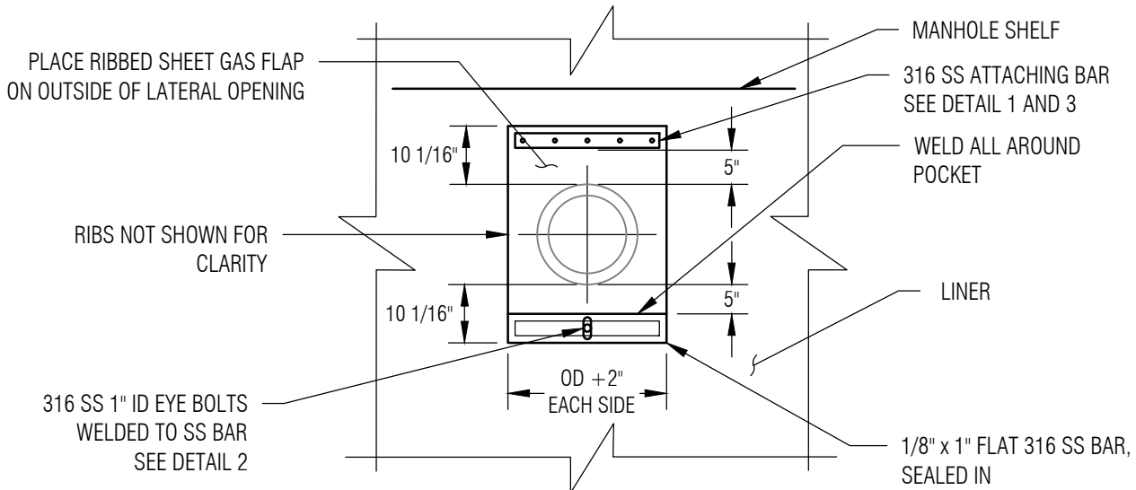
ELEVATION B
